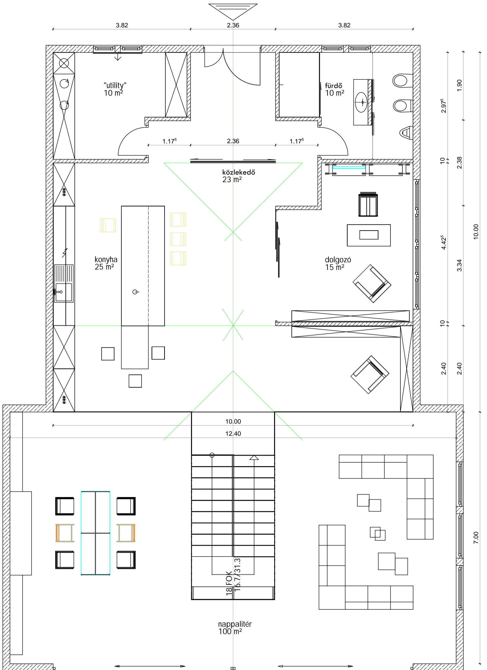
LAKÓTÉR KIALAKÍTÁSA SZABAD BRIEF ALAPJÁN - FSZ./FUNKCIONÁLIS TÉRSZERV. / 2016.05. / M= 1:50
